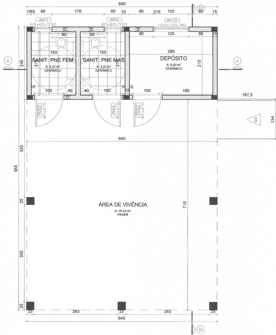
Planta baixa arquitetônico Esc:1/75
