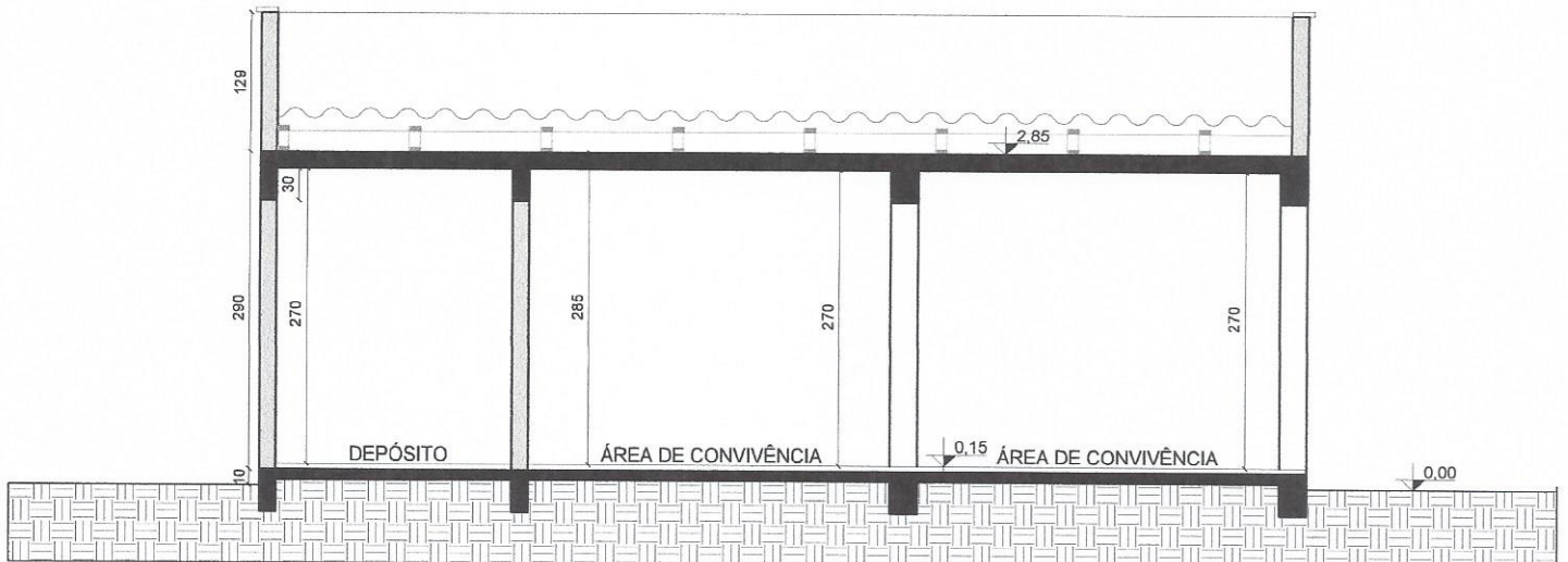
Corte B'B Esc:1/75
