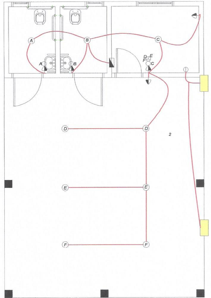
Planta elétrica Esc:1/75
