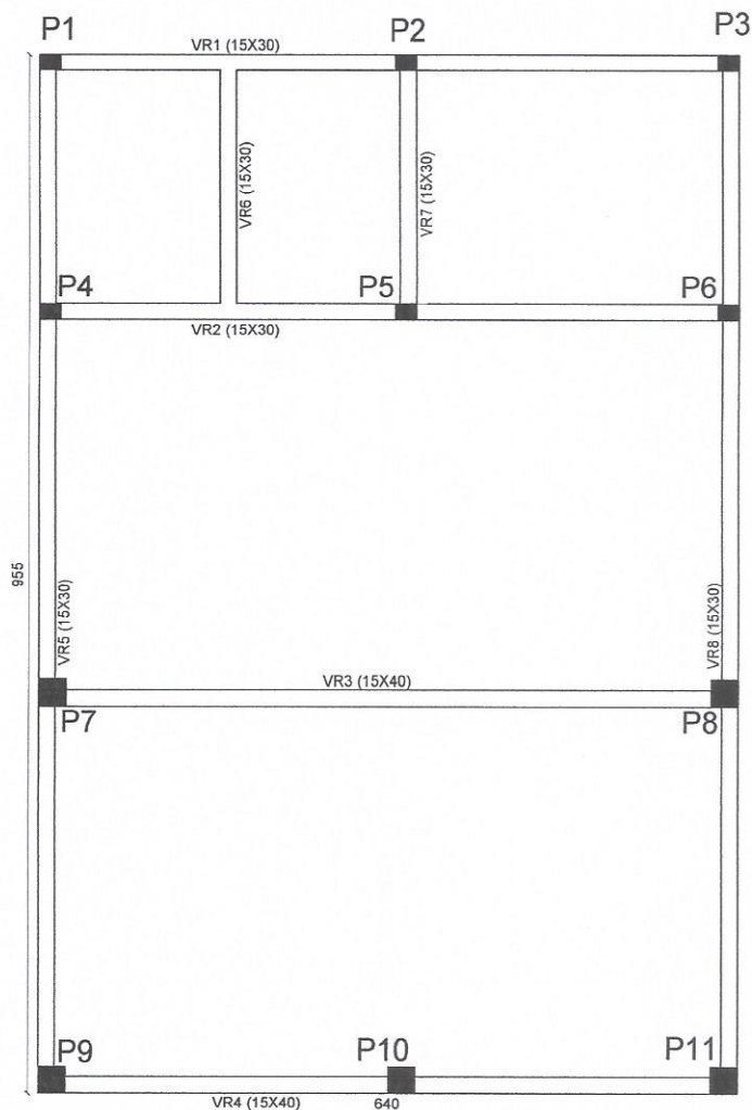
Planta estrutural vigas respaldo Esc:1/75
