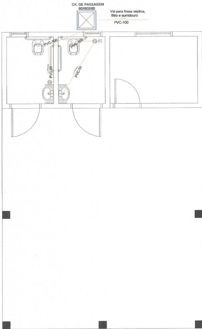
Planta de esgoto Esc:1/75
