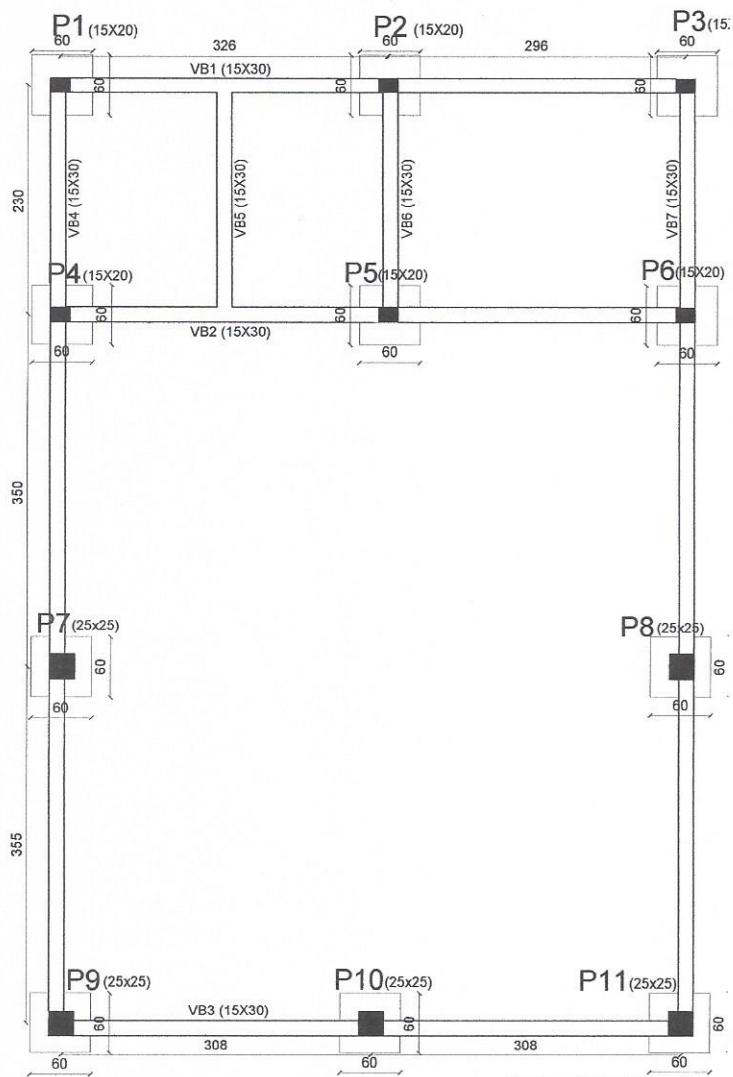
Planta estrutural fundação Esc:1/75
