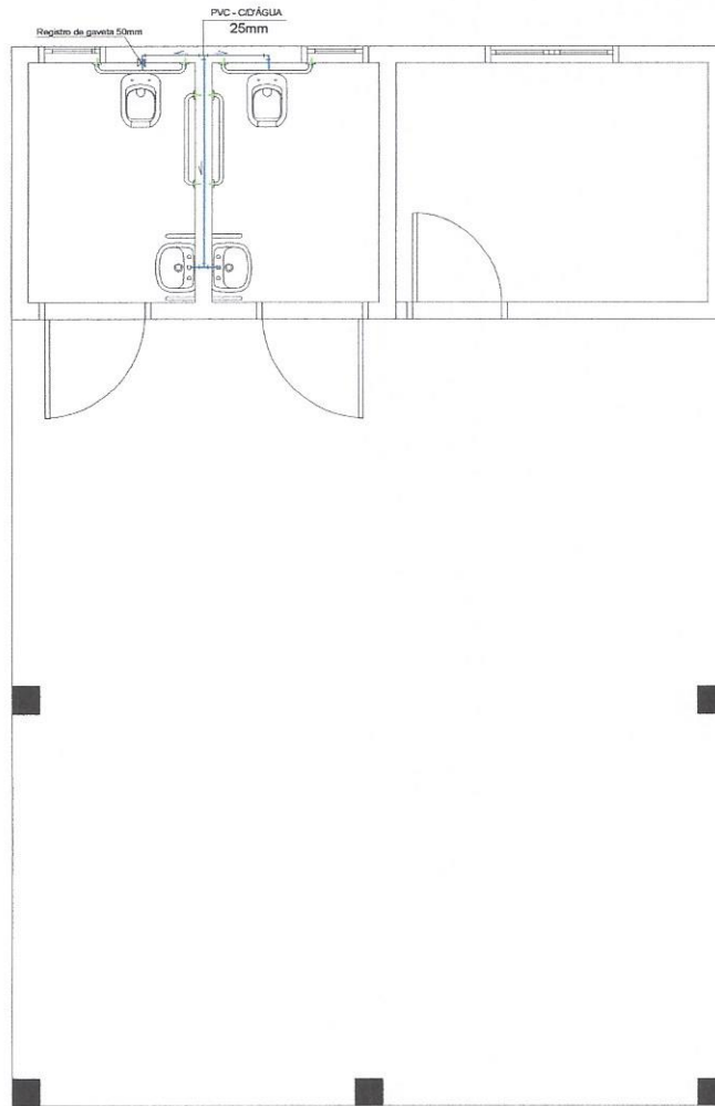
Planta de água fria Esc:1/75
